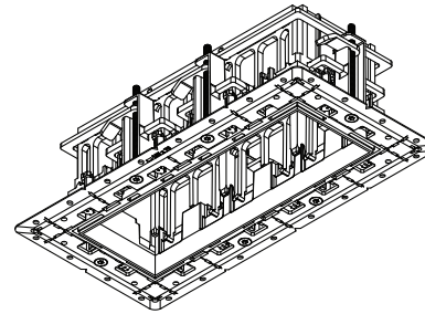
Qbini trimless frame 3x (141802XX)
